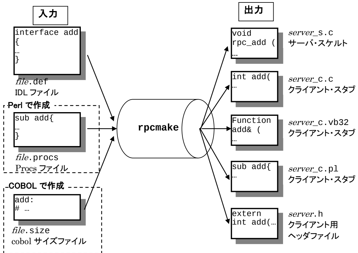
図 6.4 : RPCMake の関連ファイル
