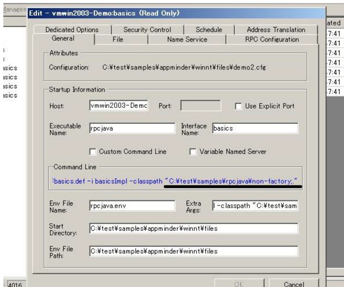
図 9.3 : AmViewer(ビューア)での「-classpath」指定の例
