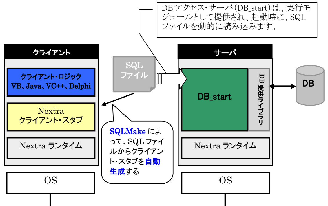
図 7.1 : DB アクセス・サーバの使用
