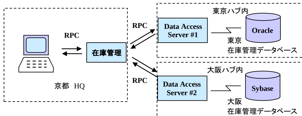
図 2.3 : データパスの例
