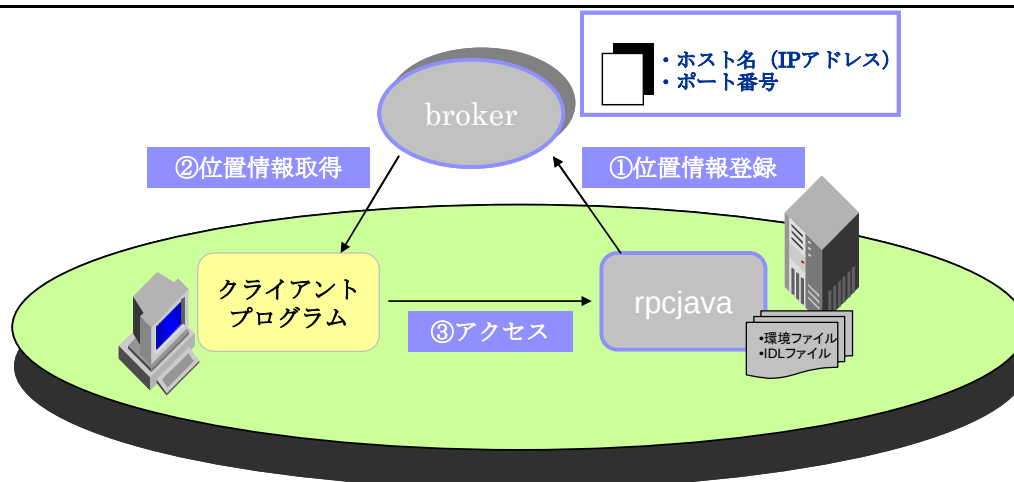
図 9.2 : rpcjava 稼動イメージ
