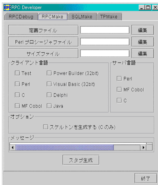
図 6.2 : RPCMake の GUI 画面
