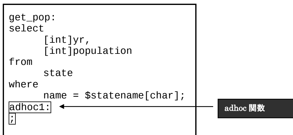
図 8.2 : SQL ファイルの adhoc 関数
