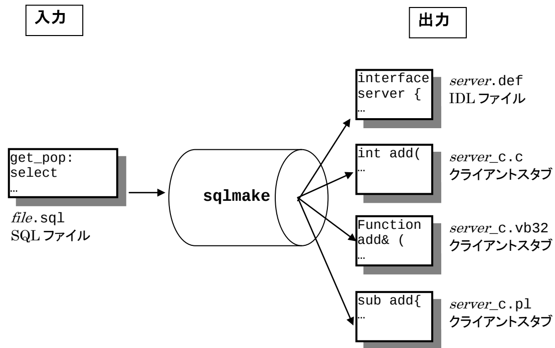
図 8.4 : SQLMake の関連ファイル
