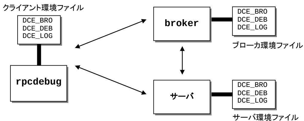
図 6.5 : サーバのテストのための構成
