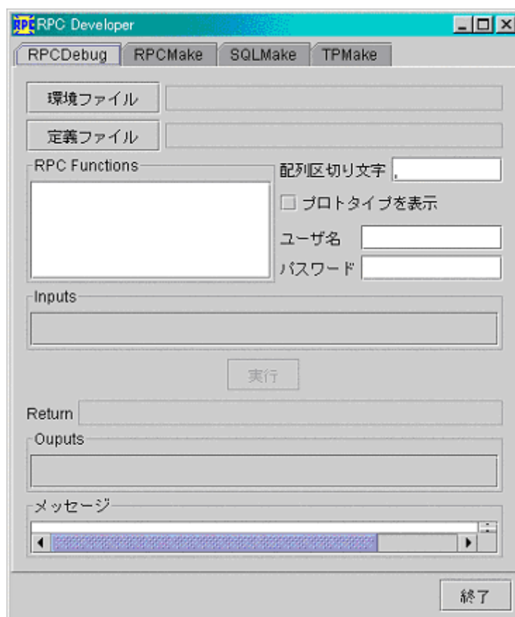
図 6.6 : RPCDebug の GUI 画面
