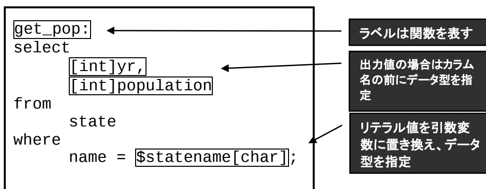
図 8.1 : 関数ラベル、引数変数、データ型指定の例
