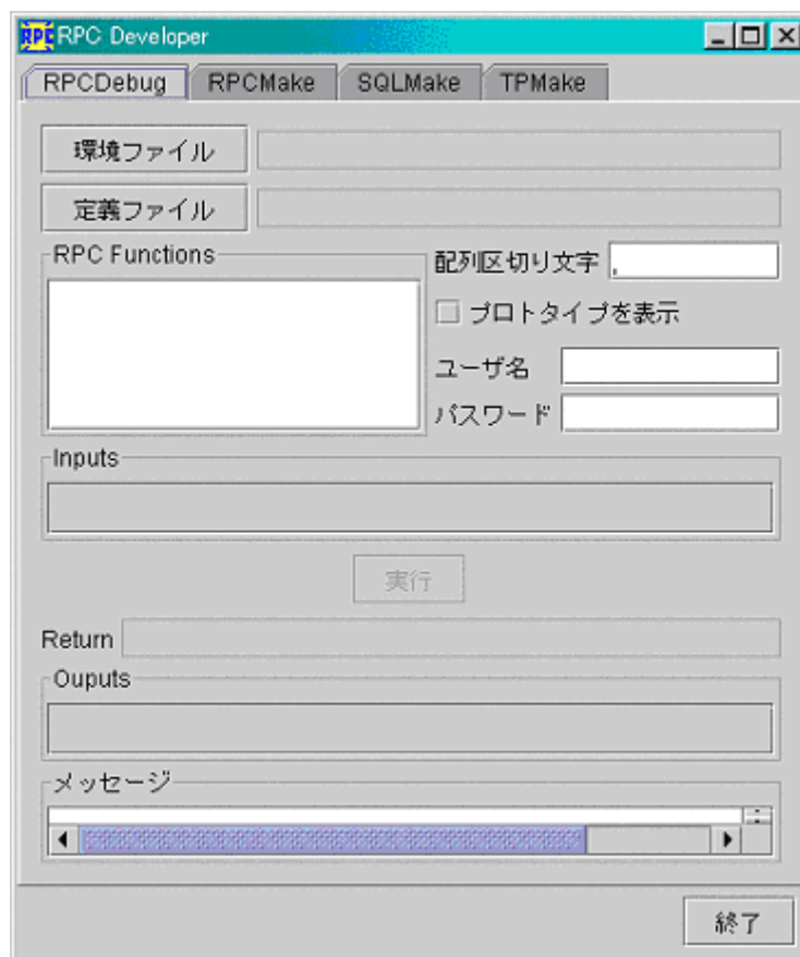
図 3.1 : RPCDebug メインウィンドウ
