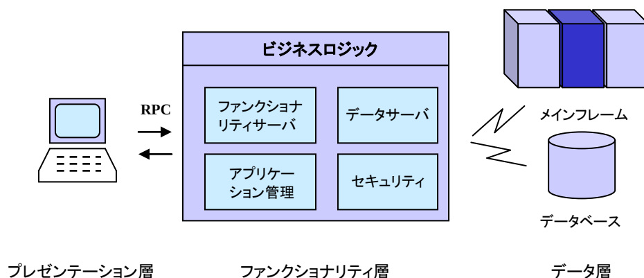
図 2.2 : 3 層構造アーキテクチャ
