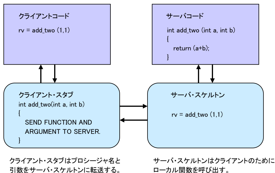
図 2.1 : リモート関数呼び出し
